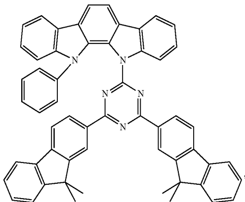
Compound E12
