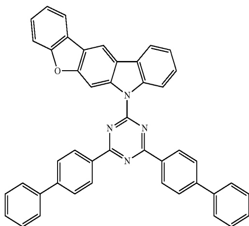
Compound E36
