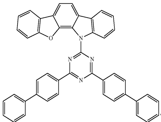
Compound E13 5
