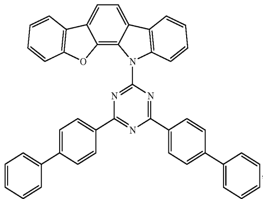
Compound E14
