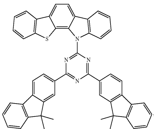
Compound E14
